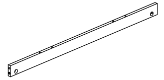
4 (768x45x12mm x1)
