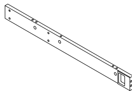
5 (798x75x23mm) X 2
